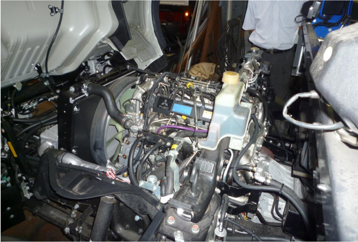
LPG とディーゼルのデュアルフューエルエンジンシステム
